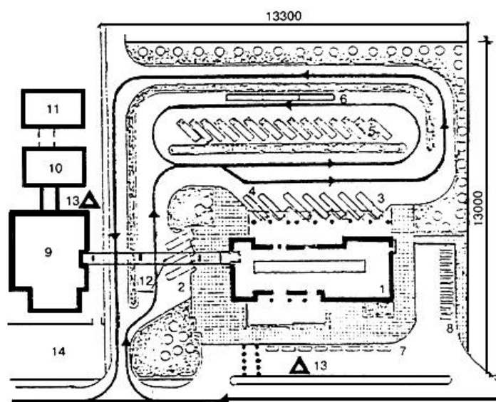
Рис. 13. Реконструкция застройки на территории общественного центра с автовокзалом
