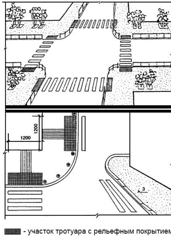
Рис. 8. Устройство переходов через внутризаводские проезды
