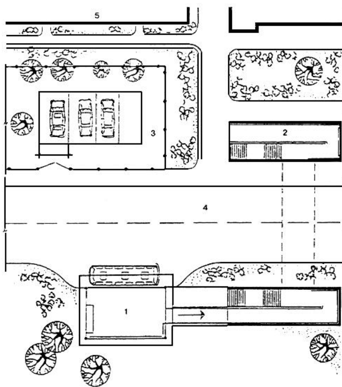
Рис. 6. Оборудование регулируемого наземного перехода для инвалидов
