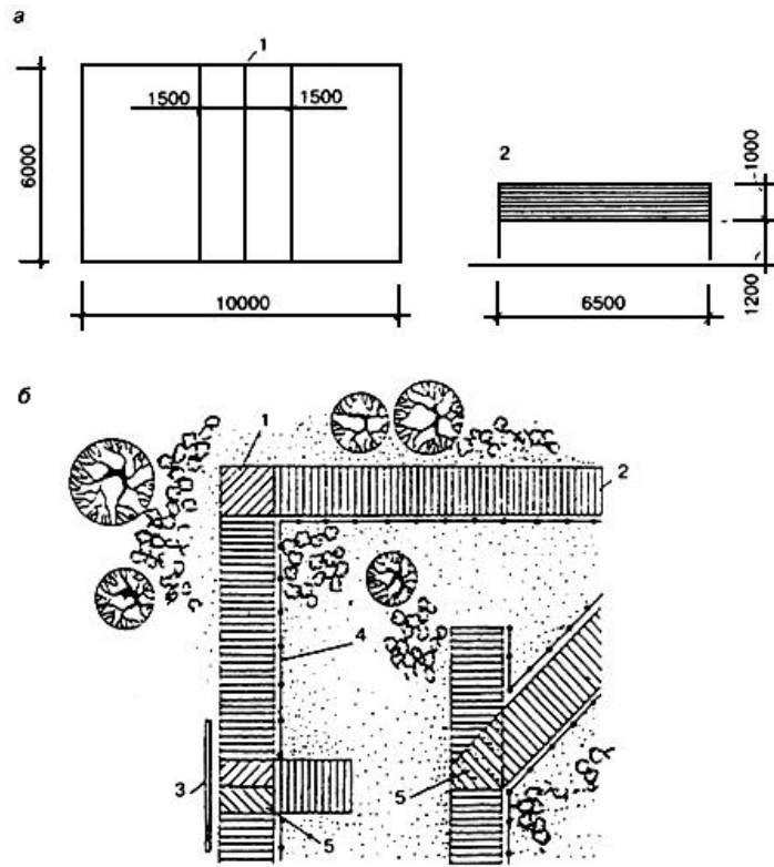
Рис. 10. Схема организации природной тропы
