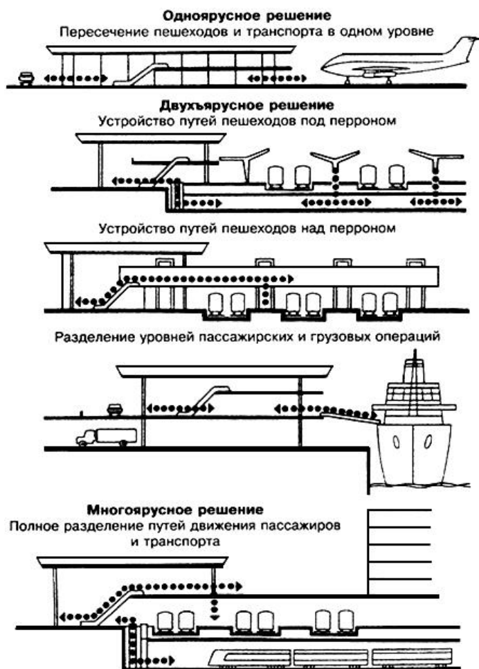
Рис. 12. Приемы организации движения пассажиров в вокзальных комплексах различного назначения
