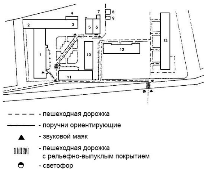
Рис. 4. Размещение ориентирующих устройств на предприятии для слепых и слабовидящих инвалидов
