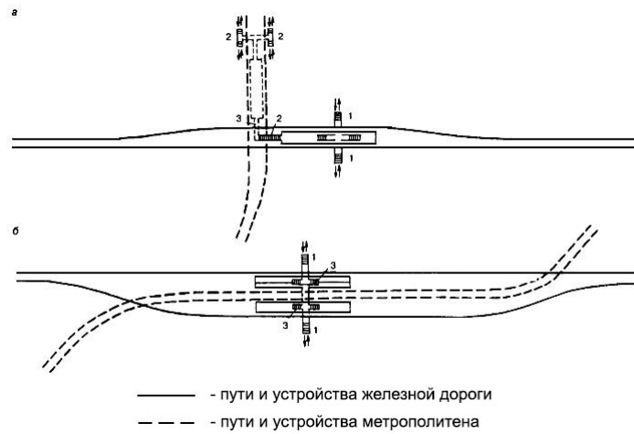
Рис. 21. Размещение остановочных пунктов взаимодействующих видов транспорта при Т-образной (а) и параллельной (б) схемах
