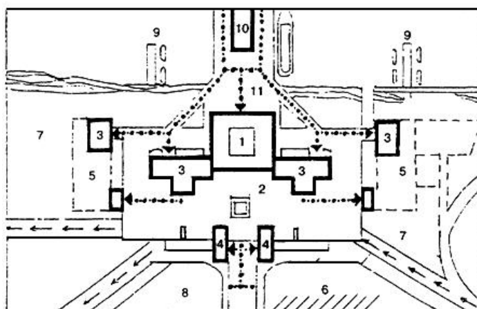
Рис. 14. Реконструкция застройки на территории общественного центра с морским вокзалом
