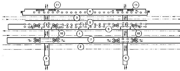
Рис. 17. Организация пересадочного узла при совмещении станций железной дороги и метрополитена с учетом потребностей инвалидов
