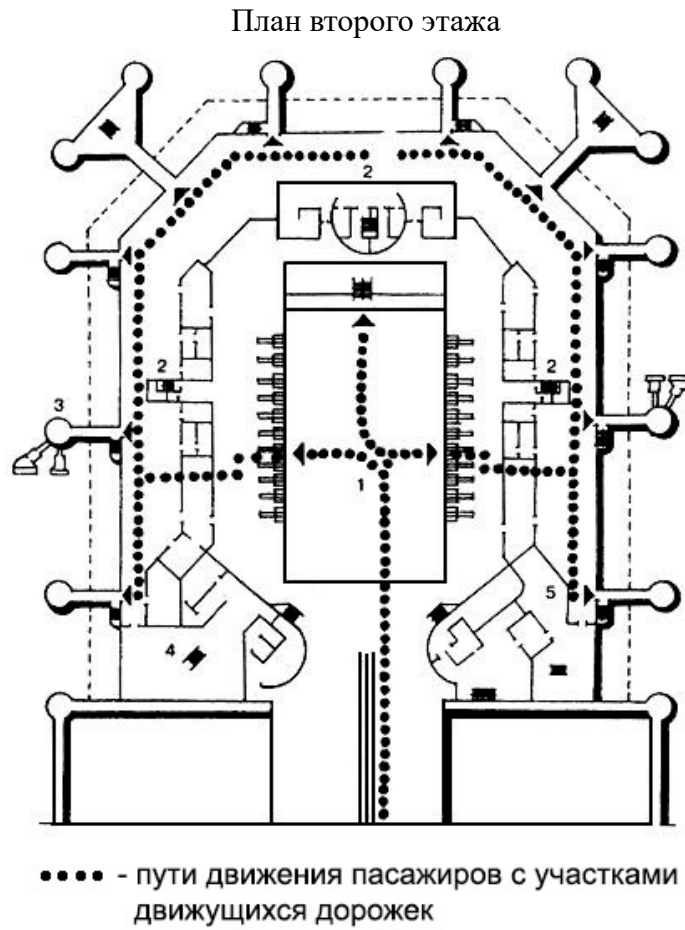
Рис. 22. Организация движения пассажиров в аэровокзале
